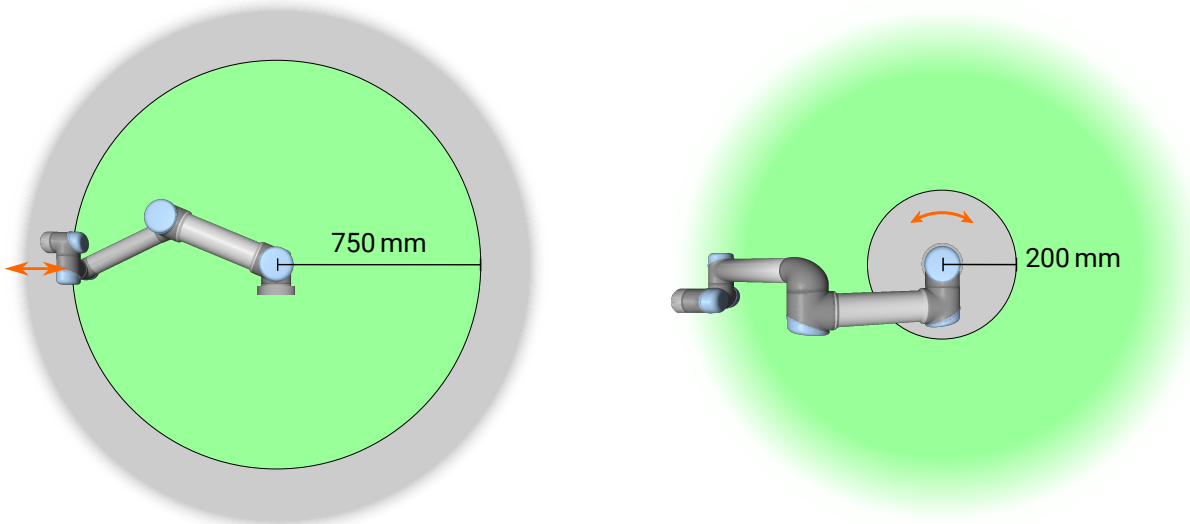
Figure 2.1: 로봇암의 물리적 특성으로 인해 특정 작업 공간 영역에서는 집히는 위험에 주의해야 한다. 리스트 1 조인트가 로봇베이스로부터 최소한 750 mm 인 경우 제한 영역 (왼쪽) 이 방사형 동작을 위해 정의된다. 접선 방향으로 움직이는 경우, 다른 영역 (오른쪽) 은 로봇베이스로부터 200 mm 거리 내에 있다.
