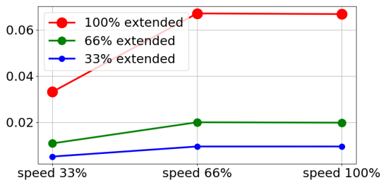
(a) 최대가반하중 33% 의미터단위정지거리
