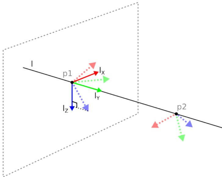
Figure 16.3: 라인특징의 정의
