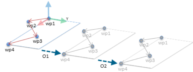
Figure 16.6: 플레인특징에오프셋을적용함
