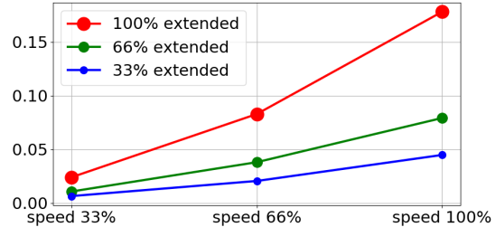
(b) 최대가반하중 66% 의미터단위정지거리
