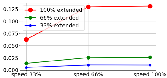
(c) 최대가반하중의정지거리미터
