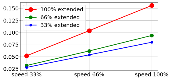
(c) 최대가반하중에대한초단위의정지시간
