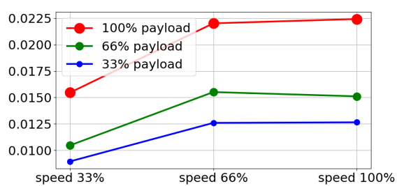
(a) Distanța de oprire în metri pentru toate încărcăturile
