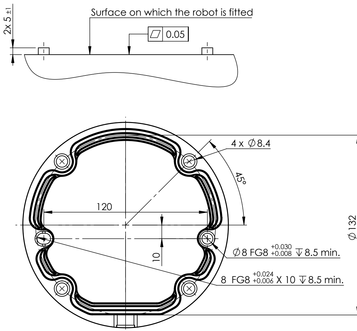
Figura 4.1: Găuri pentru montarea robotului. Utilizați patru M8 șuruburi. Toate măsurătorile sunt în mm.
