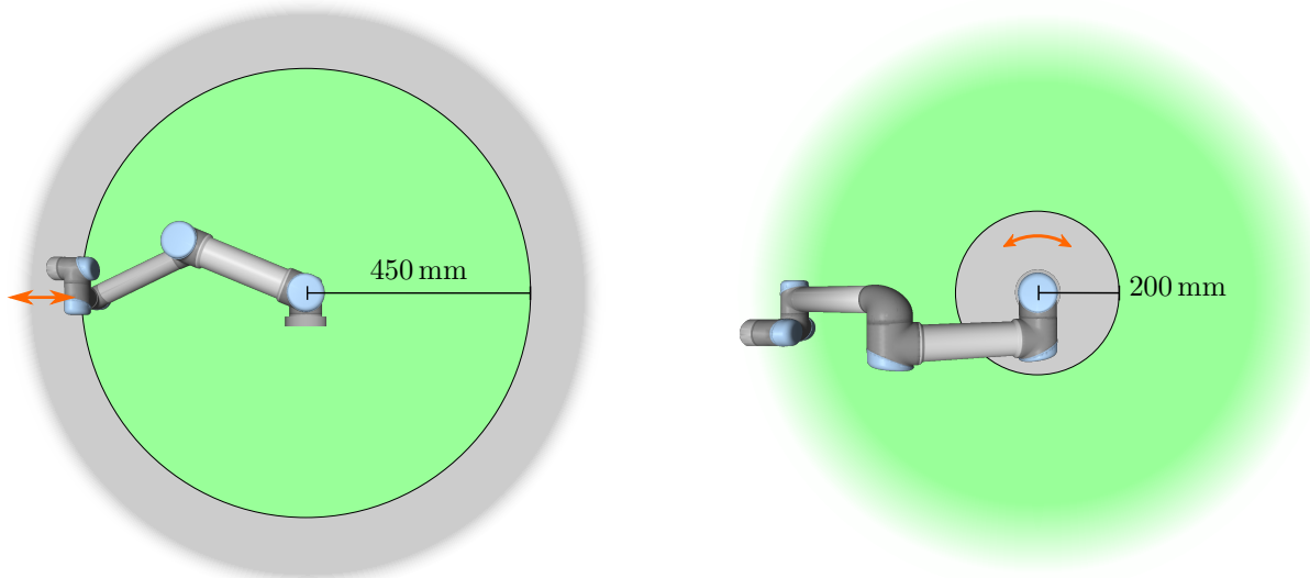
Figure 2.1: 작업영역의 특정영역은 로봇암의 물리적 특성 때문에 꼬집히는 위험을 주의해야 한다. 리스트 1 조인트가 로봇베이스로부터 최소한 450 mm 거리인 경우 한영역이 방사형 동작을 위해 정의된다. 접선 방향으로 움직이는 경우, 다른영역은 로봇베이스로부터 200 mm 거리내에 있다.
