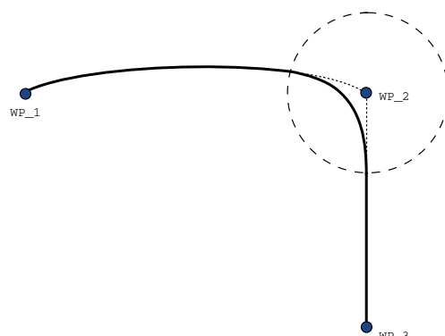
Rysunek 14.7: Przejście z ruchu w przestrzeni przegubów (RuchJ) do liniowego ruchu narzędzia (RuchL).
