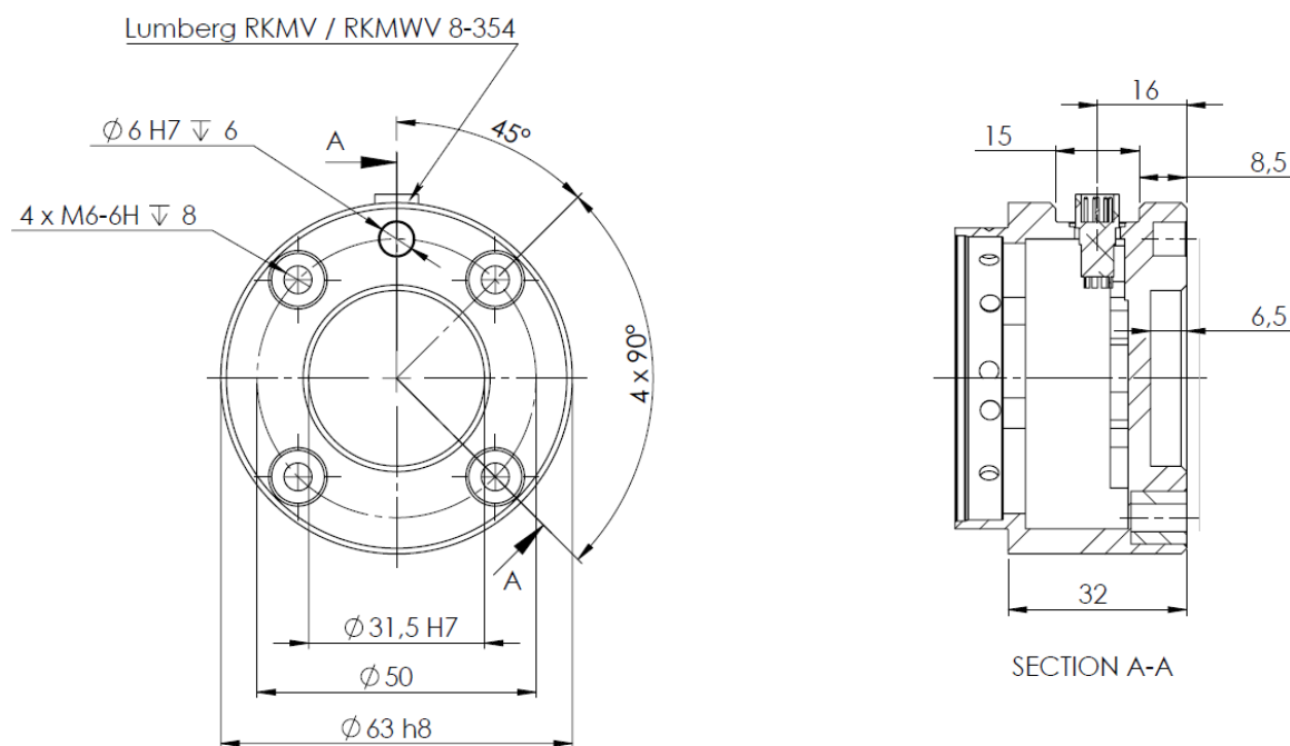
Obr. 4.2: Výstupná nástrojová prírubá, ISO 9409-1-50-4-M6. Tu sa montuje nástroj na špičku robota. Všetky miery sú v mm.
