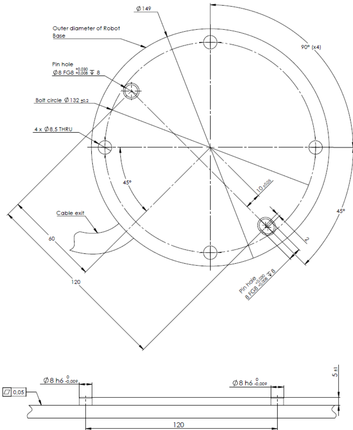
Figure 4.1: Отверстия для монтажа робота. Используются четыре M8 болта. Все измерения приведены в мм.
