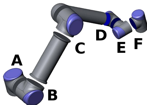
Figure 11.1: Сочленения робота. А: Основание, В: Плечевое сочленение, С: Локтевое сочленение и D, E, F: Запястье 1, 2, 3
