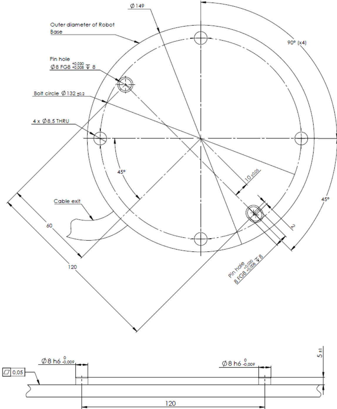
Şekil 4.1: Robotun montaj delikleri. Dört M8 cıvatası kullanın. Bütün ölçümler mm cinsindendir.
