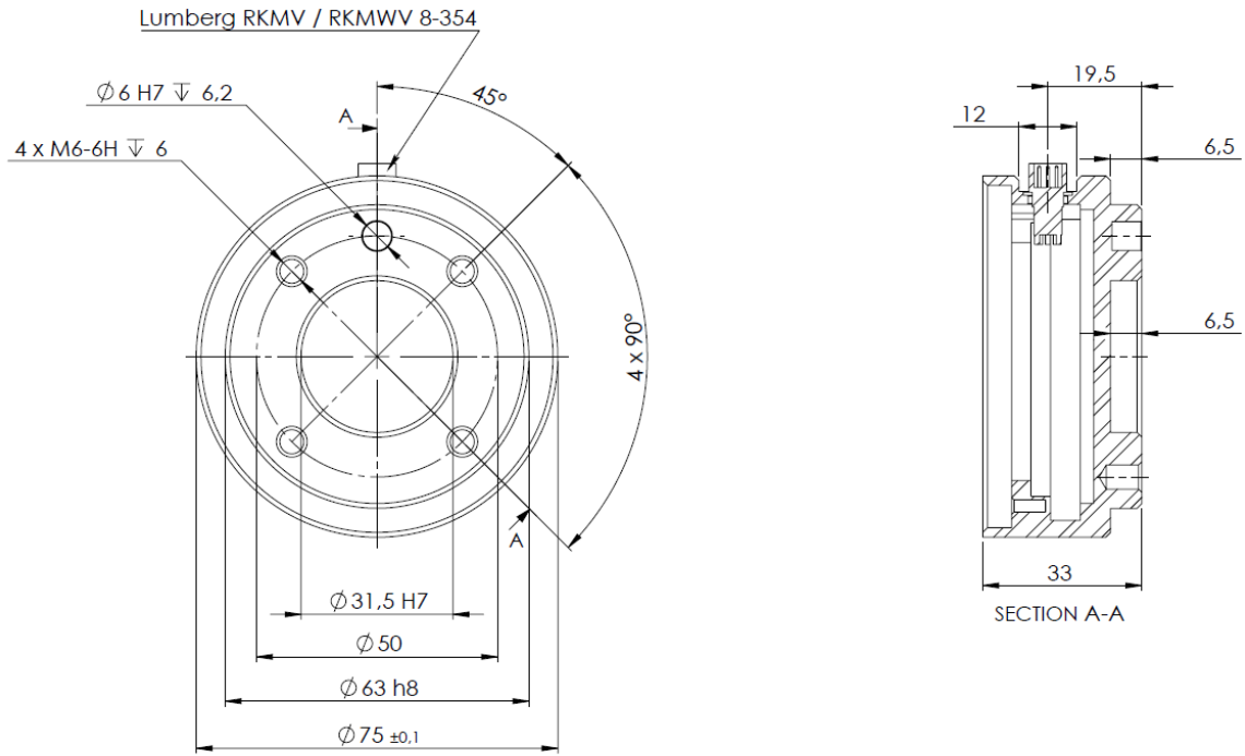
Şekil 4.2: Araç çıkış tablası, ISO 9409-1-50-4-M6. Burası, robotun uç kısmında aracın takıldığı yerdir. Bütün ölçüler mm cinsindendir.
