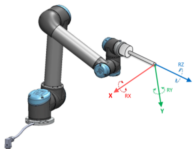
图 13.2: 工具 (TCP) 特征
