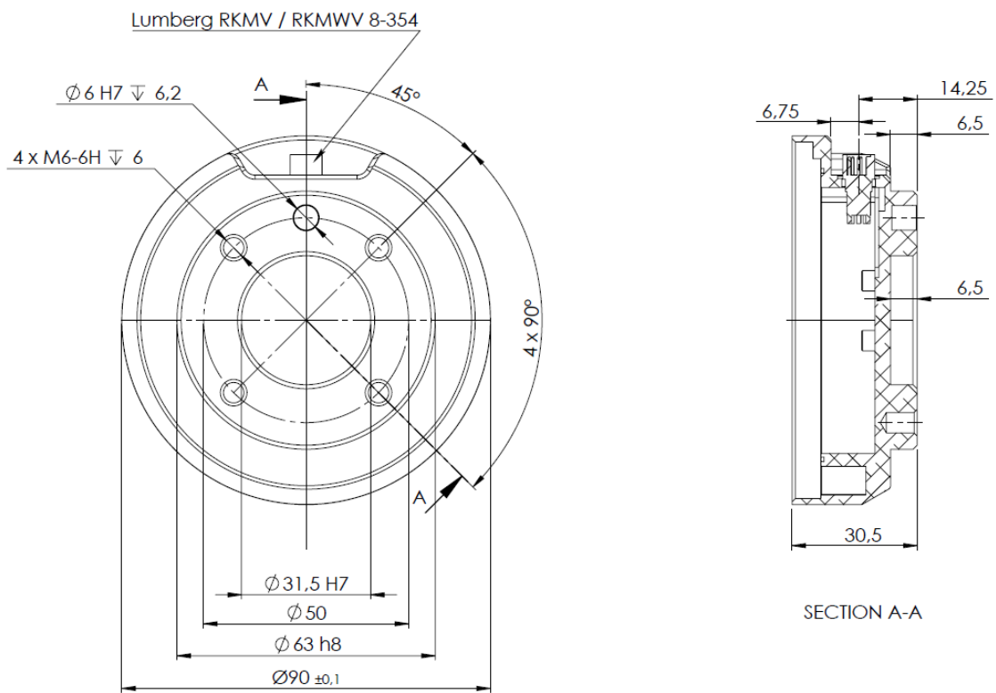
Figure 4.2: 토크출력플렌지, ISO 9409-1-50-4-M6. 여기가로봇끝에서툴을마운트하는위치이다. 모든측정 단위는 mm 이다.
