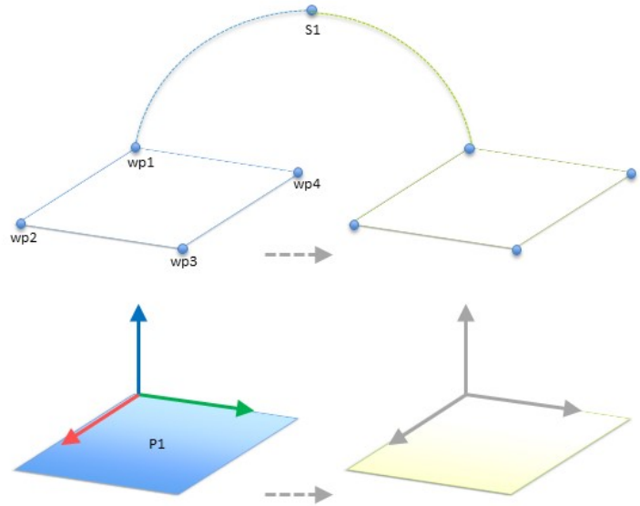
Figure 13.4: 특징변경으로수동업데이트되는특징면에대하여상대적인네개의웨이포인트를가진간단한 프로그램
