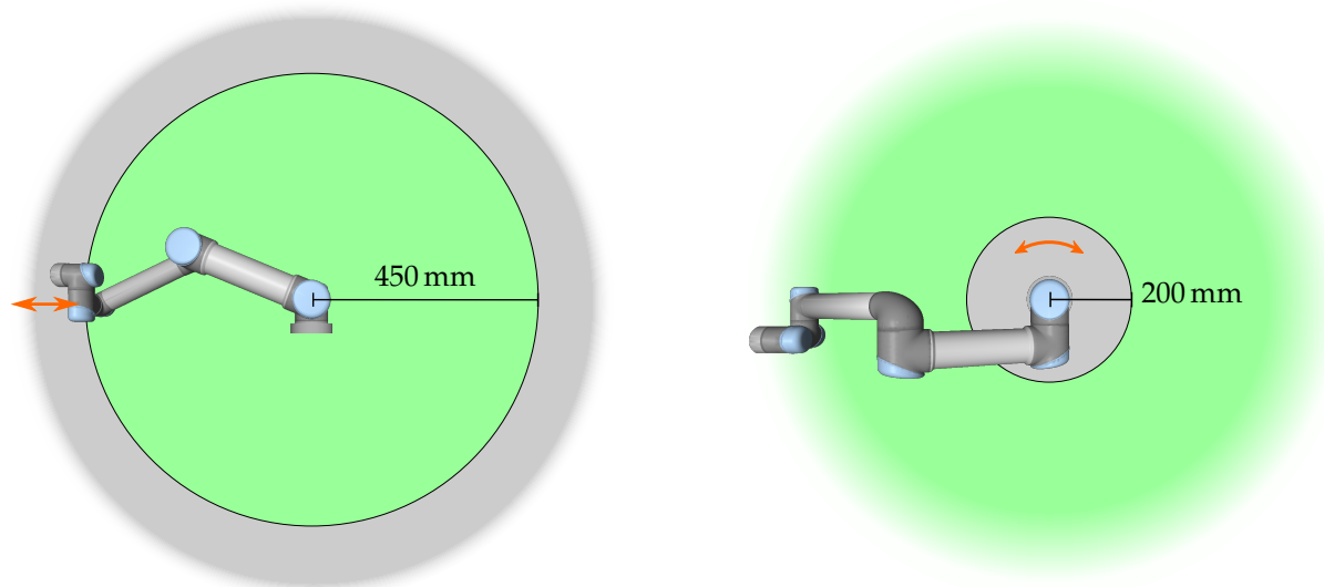
Figur 2.1: Spesielle områder til arbeidsplassen bør få oppmerksomhet angående klemmefare, som følge av robotarmens fysiske egenskaper. Et område defineres for radiale bevegelser, når handleddd 1-leddet er på en avstand på minst 450 mm fra basen til roboten. Det andre området er innen 200 mm fra basen til roboten, når den beveger seg i den tangentielle retningen.
