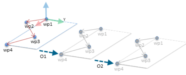
FIGURE 13.6 – Appliquer un décalage à la fonction de plan
