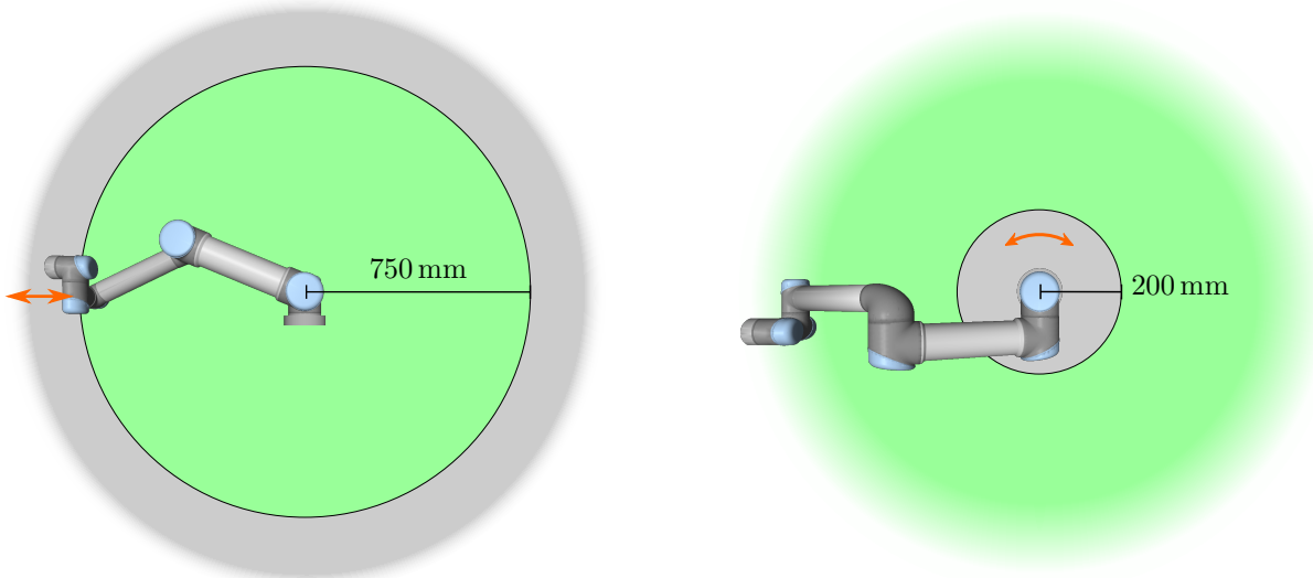
Figure 2.1: 작업영역의 특정영역은 로봇암의 물리적 특성 때문에 꼬집히는 위험을 주의해야 한다. 손목 1 조인트가 로봇베이스로부터 최소한 750 mm 거리인 경우 한 영역이 방사형 동작을 위해 정의된다. 접선 방향으로 움직이는 경우, 다른 영역은 로봇베이스로부터 200 mm 거리 내에 있다.
