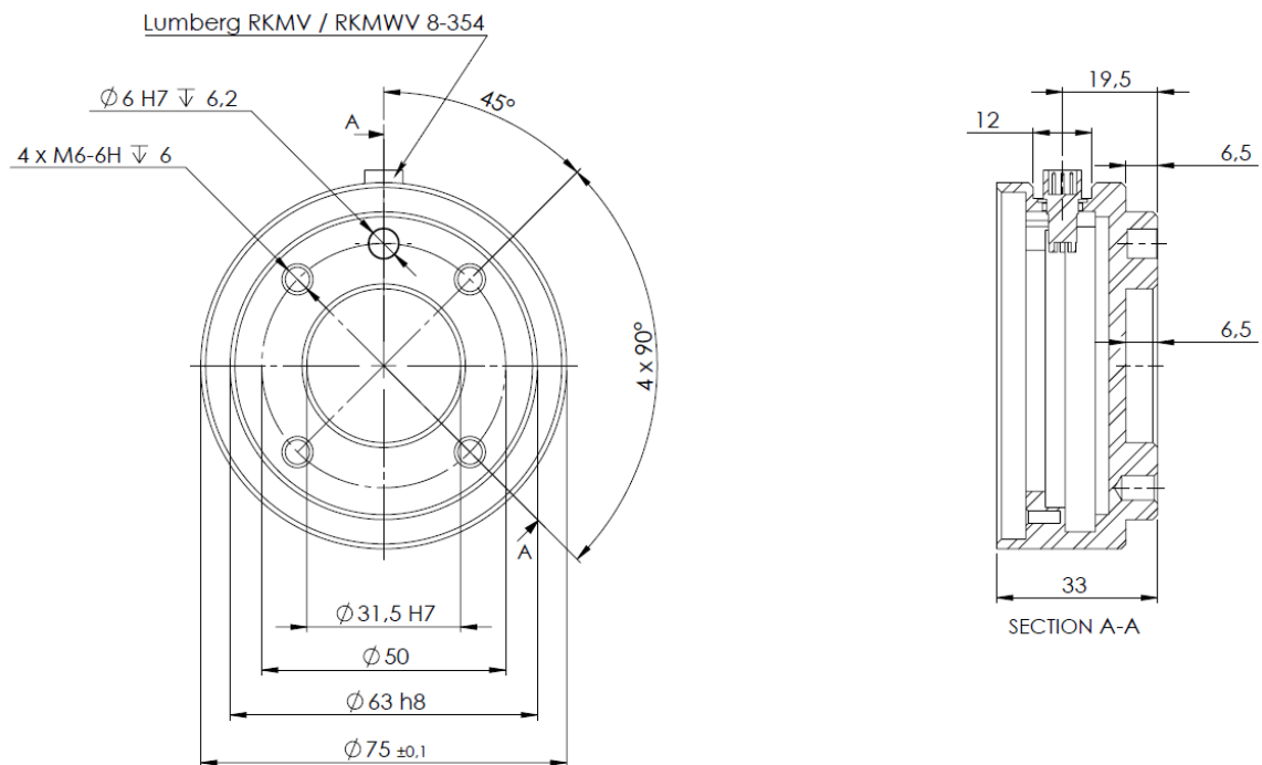
Figure 4.2: 토크출력플렌지, ISO 9409-1-50-4-M6. 여기가로봇끝에서툴을마운트하는위치이다. 모든측정 단위는 mm 이다.
