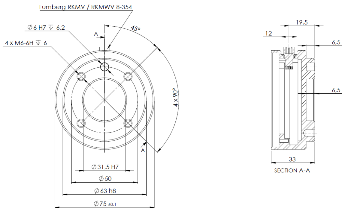
Figure 4.2: Фланец для подсоединения инструмента, ISO 9409-1-50-4-M6. В этом месте инструмент прикрепляется к наконечнику робота. Все измерения приведены в мм.
