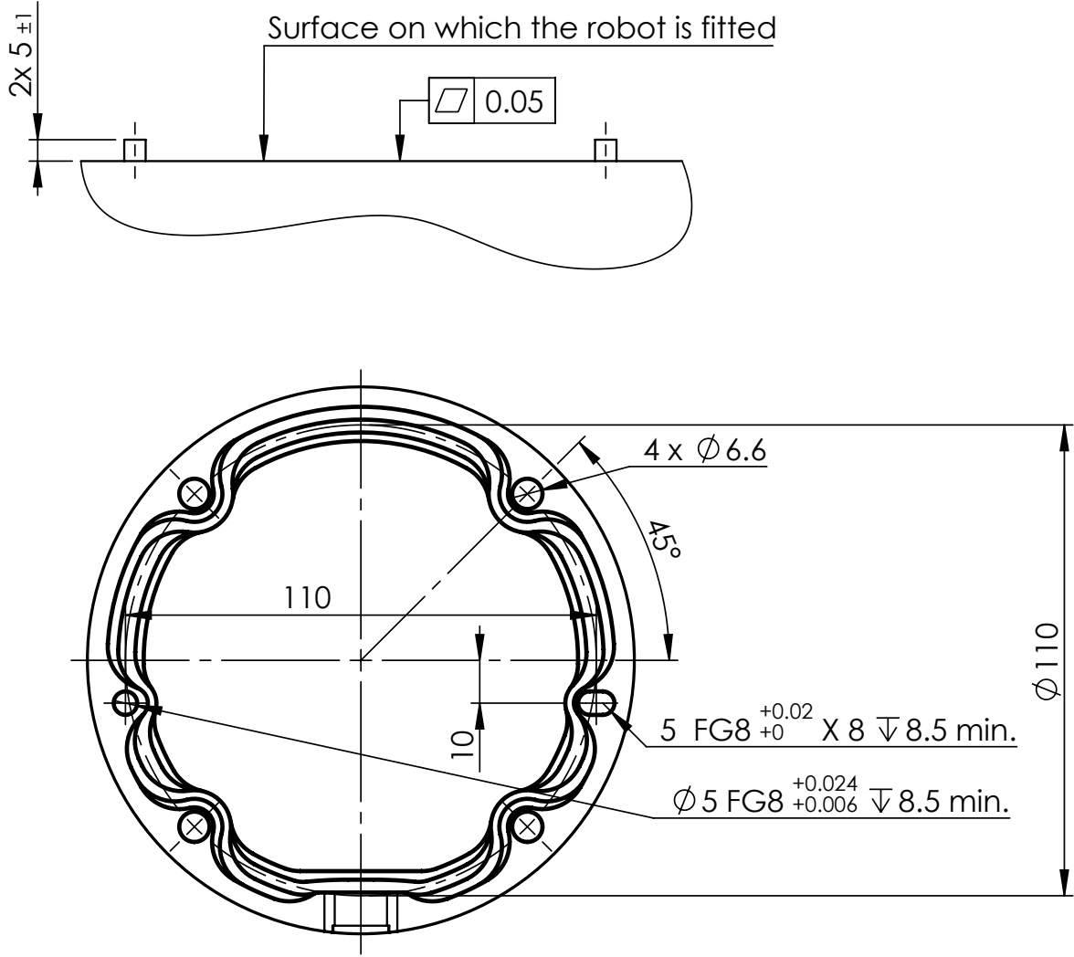
Şekil 4.1: Robotun montaj delikleri. Dört M6 cıvatası kullanın. Bütün ölçümler mm cinsindendir.
