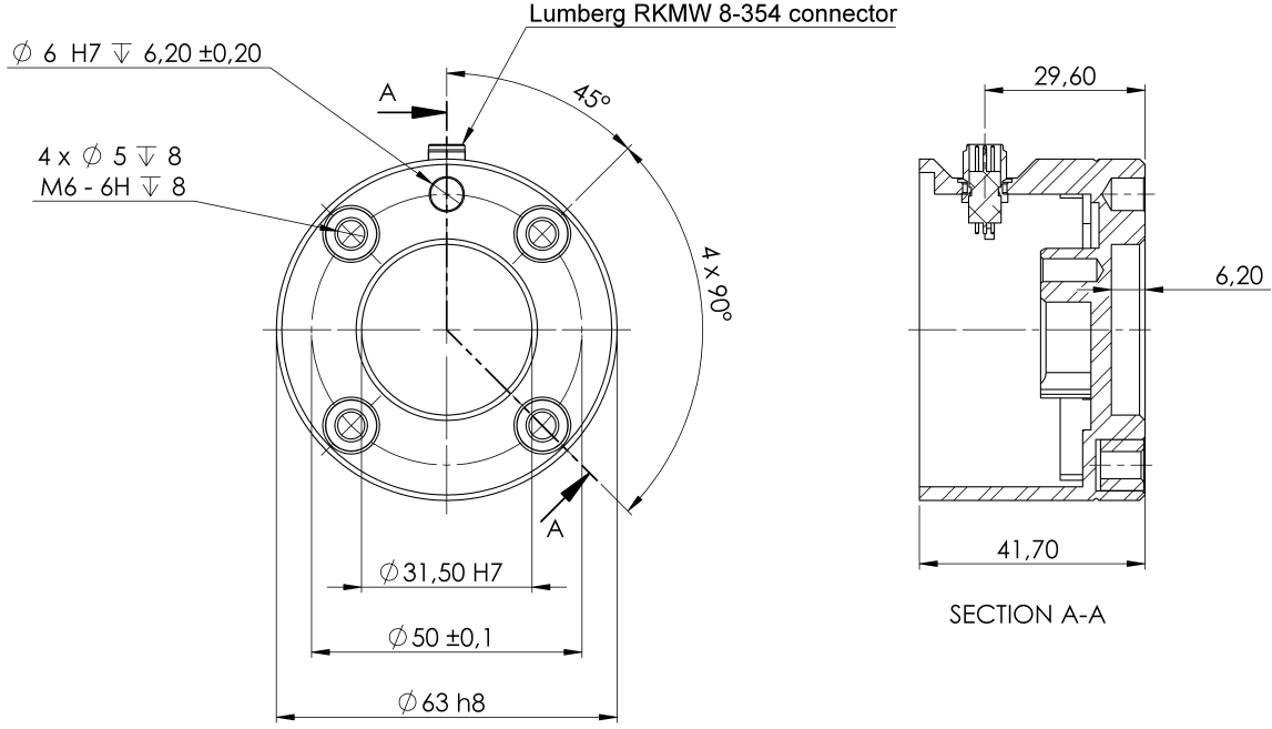
Şekil 4.2: Aletin çıkış flanşı (ISO 9409-1-50-4-M6), aletin robotun ucuna takıldığı yerdir. Bütün ölçüler mm cinsindendir.
