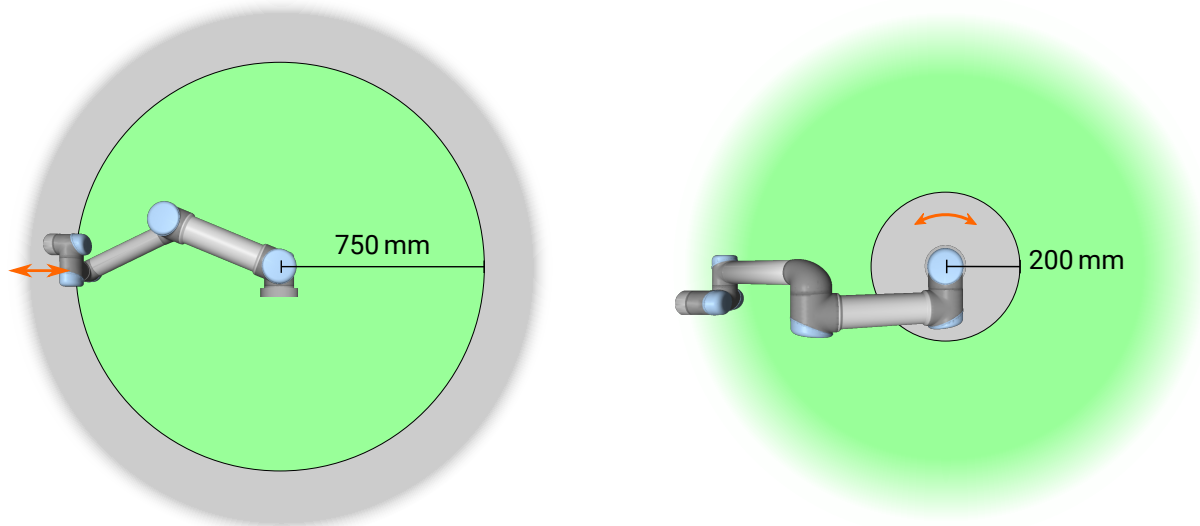
图 2.1: 由於機械手臂的物理特性，某些工作空間區域需要注意捏造危險。其中一個區域（左）是定義的徑向運動區域，即手腕 1 關節至少與機器人底座相距 750 mm 的區域。另一個區域（右）是在機器人底座 200 mm 範圍內的區域（機器人按正切方向移動時）。
