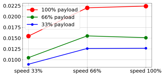
(a) 全有効荷重に対する停止距離 (メートル)
