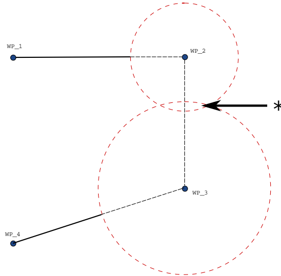
Şekil 15.4: Harman radius çakışmasına izin verilmez (*).
