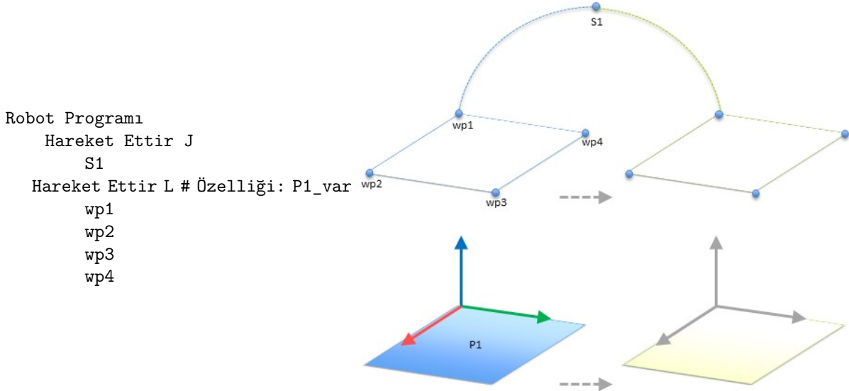
Şekil 16.4: Özellik değiştirilerek manuel olarak güncellenen bir özellik düzlemine göre dört geçiş noktalı basit program
