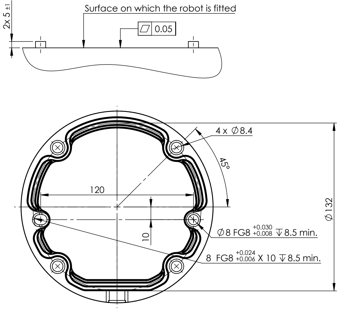
Şekil 4.1: Robotun montaj delikleri. Dört M8 cıvatası kullanın. Bütün ölçümler mm cinsindendir.
