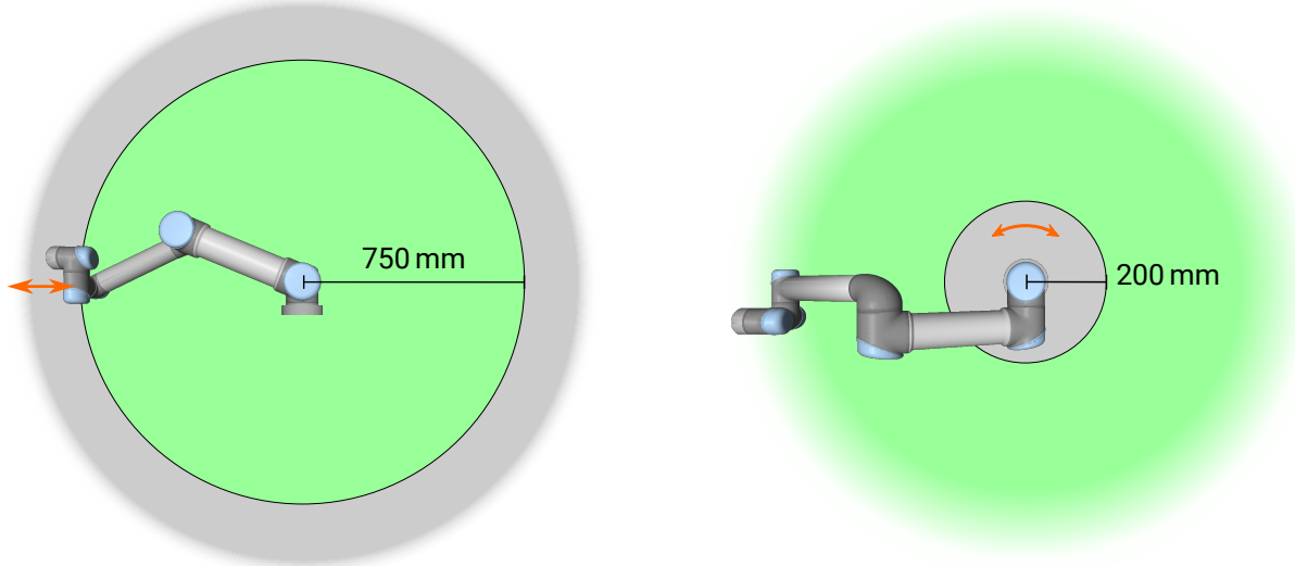
Şekil 2.1: Robot kolunun fiziksel özelliklerinden dolayı, bazı çalışma alanlarına sıkıştırma tehlikeleriyle ilgili olarak dikkat edilmesi gerekir. Bilek 1 eklemiyle robot tabanı arasında en az 750 mm olduğunda, radyal hareketler için bir alan (sol) tanımlanır. Diğer (sağdaki) alan, teğet hareket ederken robotun tabanının 200 mm yakınındadır.
