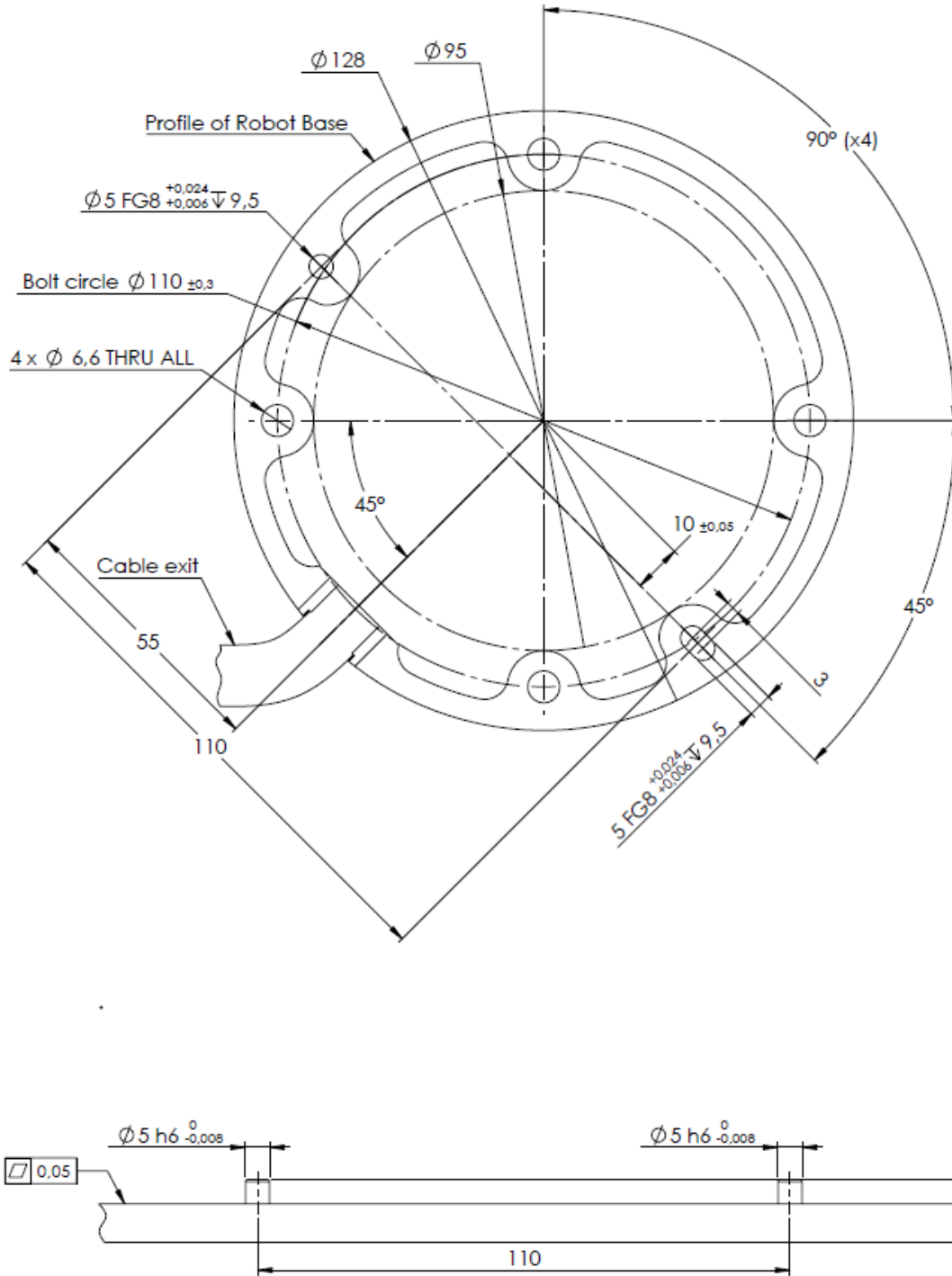
Şekil 4.1: Robotun montaj delikleri. Dört M6 cıvatası kullanın. Bütün ölçümler mm cinsindendir.
