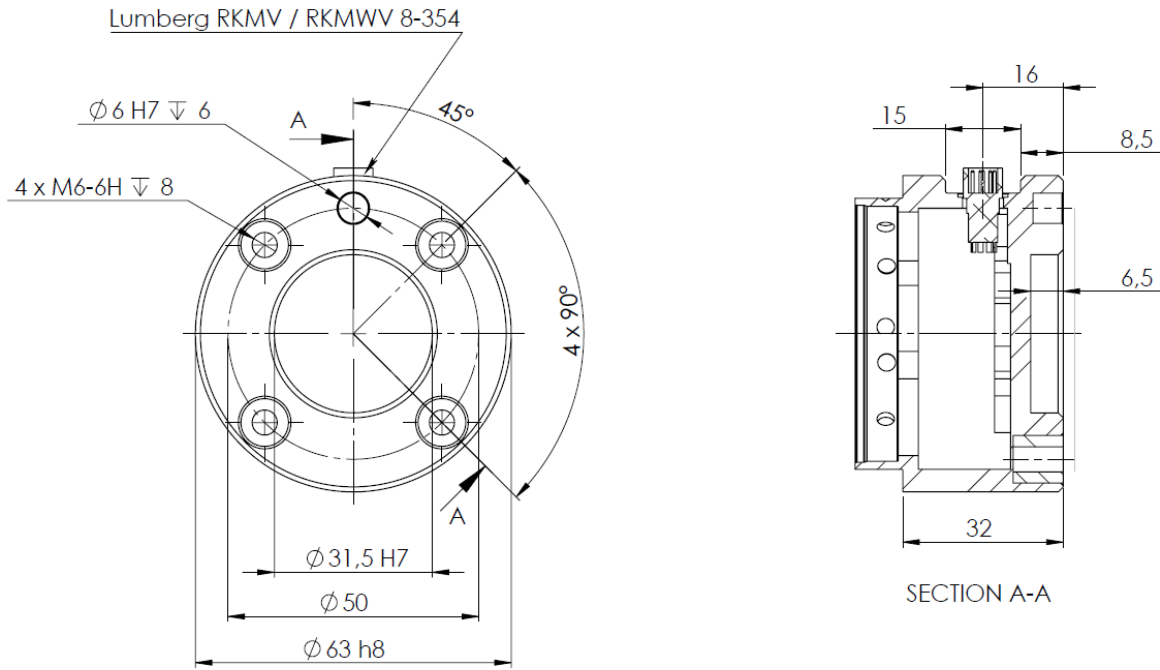
Şekil 4.2: Araç çıkış tablası, ISO 9409-1-50-4-M6. Burası, robotun uç kısmında aracın takıldığı yerdir. Bütün ölçüler mm cinsindendir.
