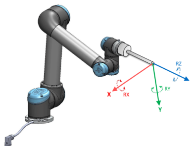
Figur 16.2: Funktionen Værktøj (TCP)
