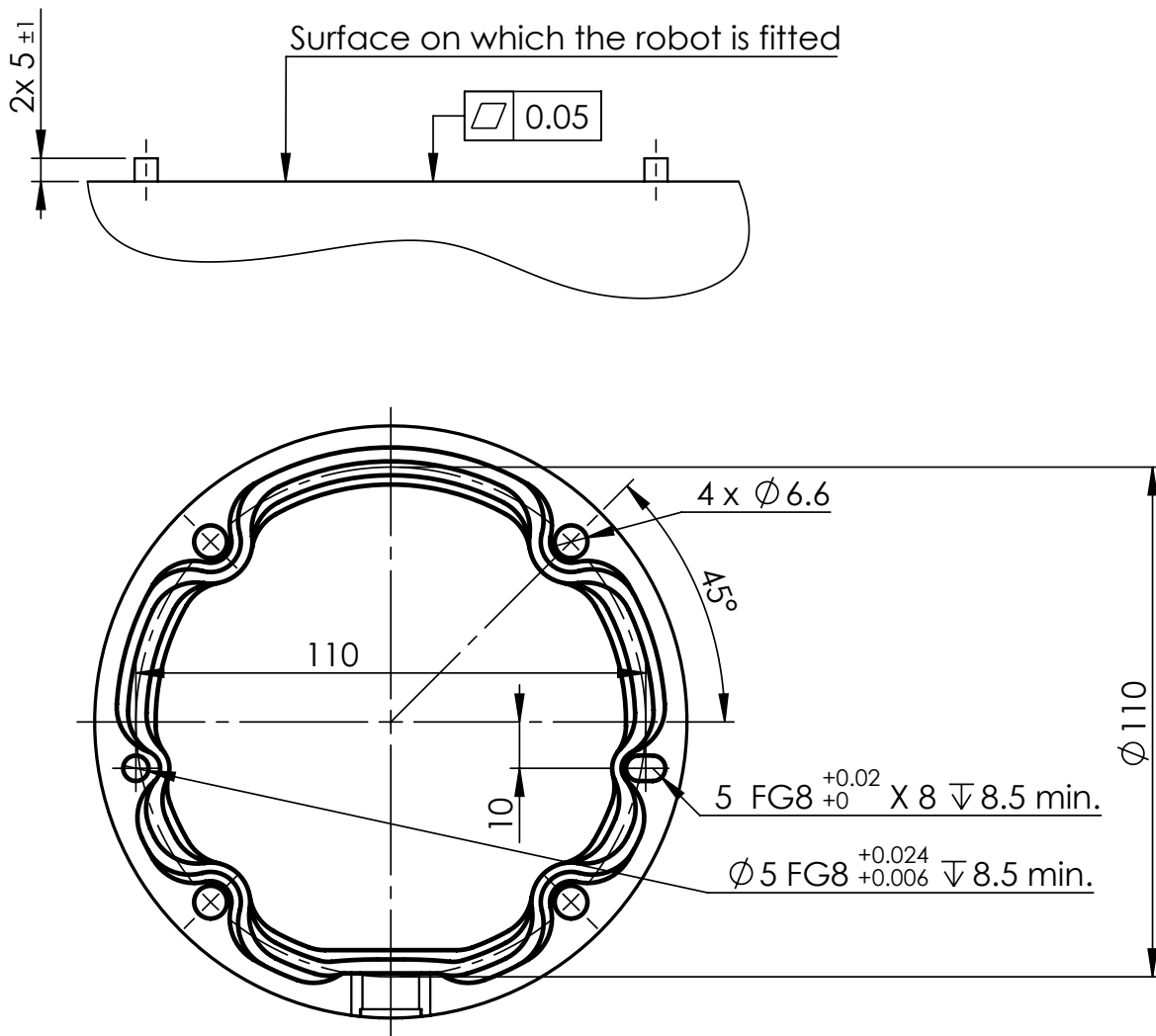
Figure 4.1: Отверстия для монтажа робота. Используются четыре М6 болта. Все измерения приведены в мм.
