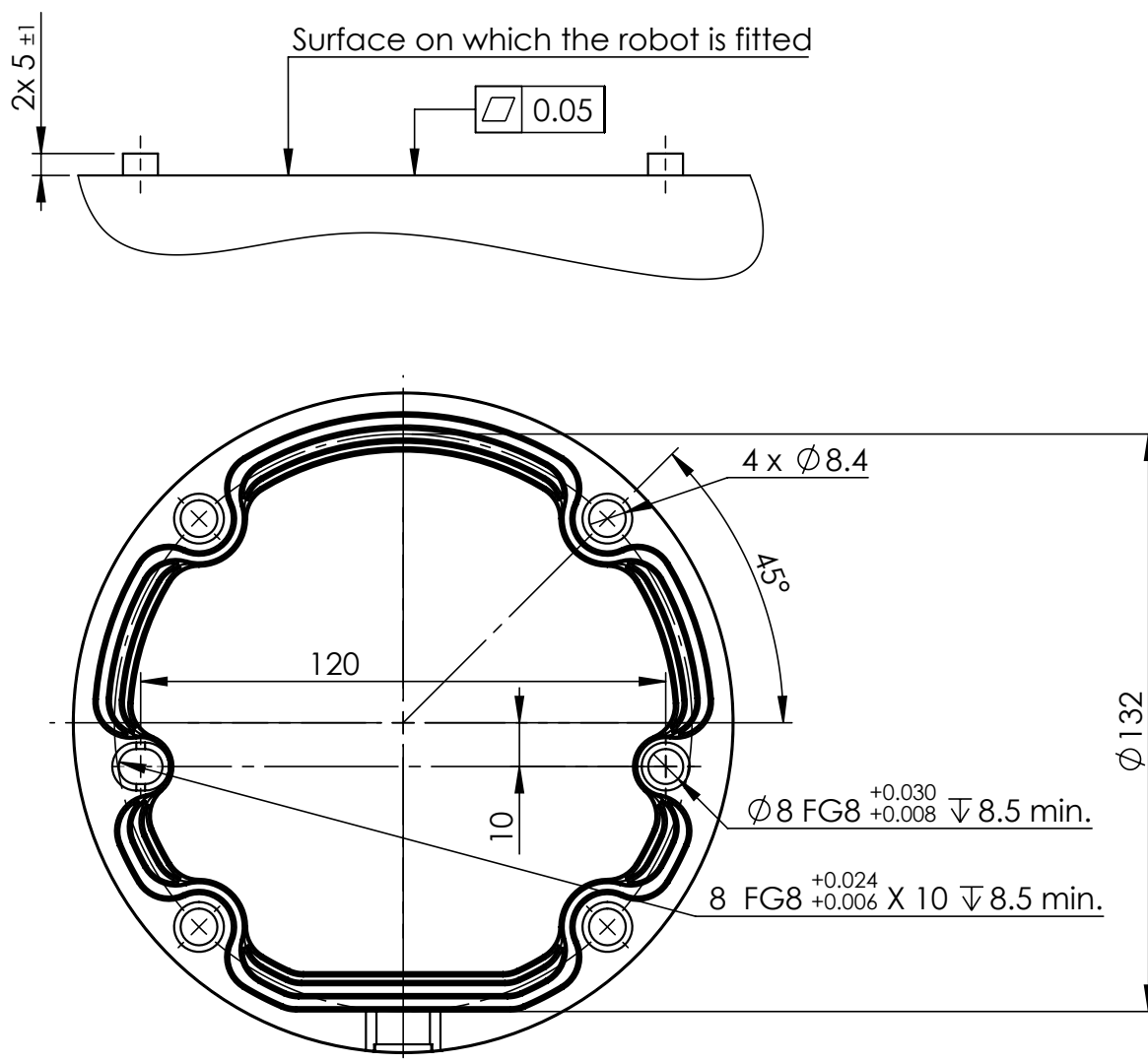
图 4.1: 機器人安裝孔。使用四個 M8 螺栓。所有測量值均以 mm 為單位。
