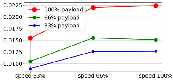
(a) Tüm taşıma kapasiteleri için metre cinsinden durdurma mesafesi
