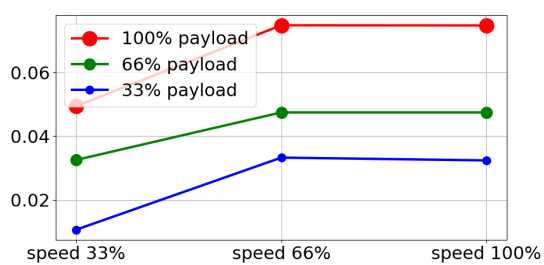
(a) Distanza di arresto in metri per tutti i carichi utili
