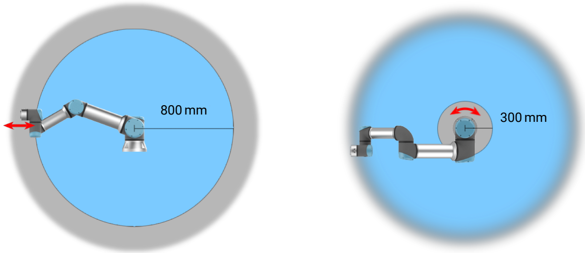
Figure 2.1: 로봇암의물리적특성으로인해특정작업공간영역에서는집히는위험에주의해야한다. 손목 1조인트가로봇베이스로부터최소한 800 mm 인경우에만영역 (왼쪽) 이방사형동작을위해정의된다. 접선방향으로움직이는경우, 다른영역 (오른쪽) 은로봇베이스로부터 300 mm 거리내에있다.
