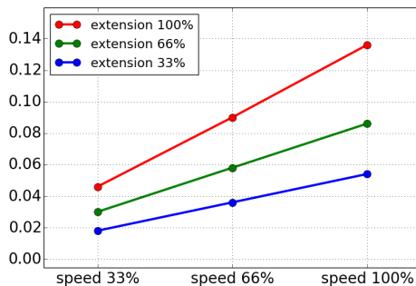
(c) Timpul de oprire în secunde pentru încărcătura maximă
