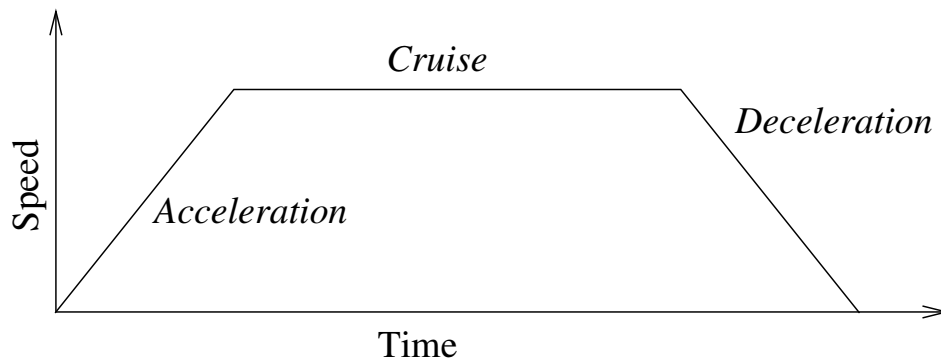
Figura 15.1: Profil viteză pentru o mișcare. Curba este împărțită în trei segmente: acclerație , croazieră și decelerație . Nivelul fazei croazieră este indicat de setarea de viteză a mișcării, în timp ce gradul de acclerație și decelerație este indicat de parametrul de accelerație.
