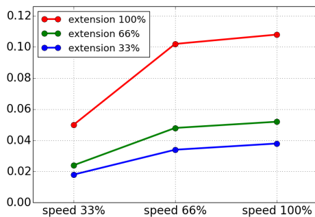
(a) Timpul de oprire în secunde pentru 33% din încărcătura maximă
