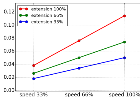
(b) Timpul de oprire în secunde pentru 66% din încărcătura maximă
