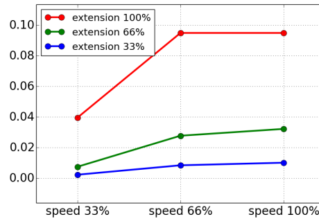
(c) Distanța de oprire în metri pentru încărcătura maximă
