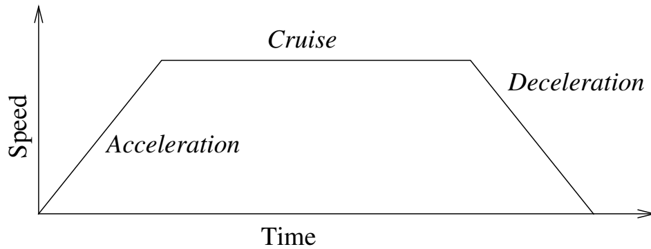
Figura 15.1: Perfil de velocidad para un movimiento. La curva se divide en tres segmentos: aceleración , cruce y desaceleración . El nivel de la fase cruce se obtiene del ajuste de velocidad del movimiento, mientras que la pendiente de las fases de aceleración y desaceleración se obtiene del parámetro de aceleración.
