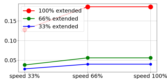
Figuur A.4: Stoptijd voor gewricht 1 (SCHOUDER)
