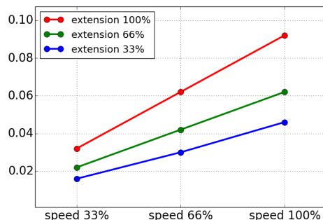
(a) Nachlaufzeit in Sekunden für 33% maximale Nutzlast
