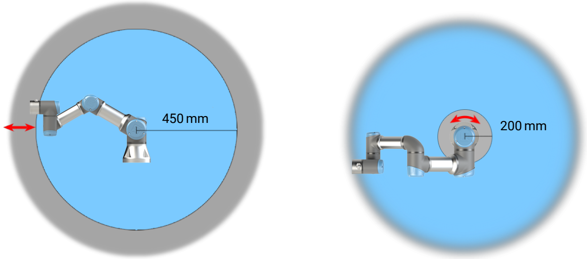
Şekil 2.1: Robot kolunun fiziksel özelliklerinden dolayı, bazı çalışma alanlarına sıkıştırma tehlikeleriyle ilgili olarak dikkat edilmesi gerekir. Bilek 1 eklemiyle robot tabanı arasında en az 450 mm olduğunda, radyal hareketler için bir alan (sol) tanımlanır. Diğer (sağdaki) alan, teğet hareket ederken robotun tabanının 200 mm yakınındadır.
