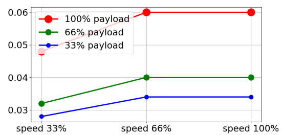
(b) Tiempo de parada en segundos para todas las cargas útiles
