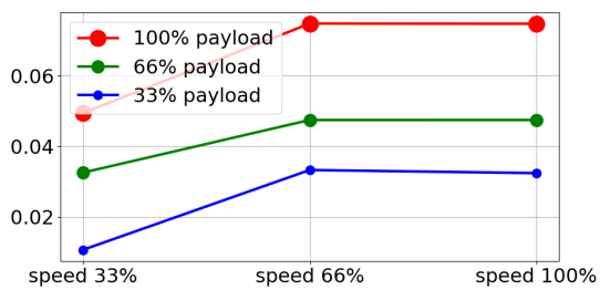
(a) 모든페이로드에대한미터단위의정지거리
