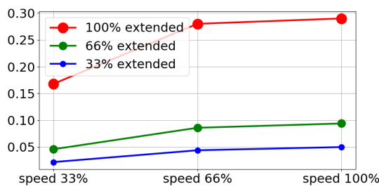
(c) 최대페이로드에대한초단위의정지시간
