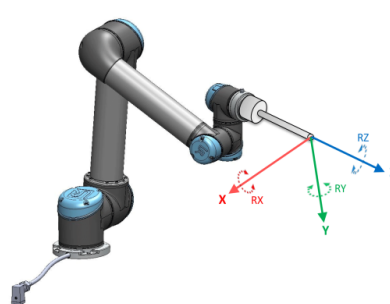
Figura 13.2: Feature utensile (TCP)
