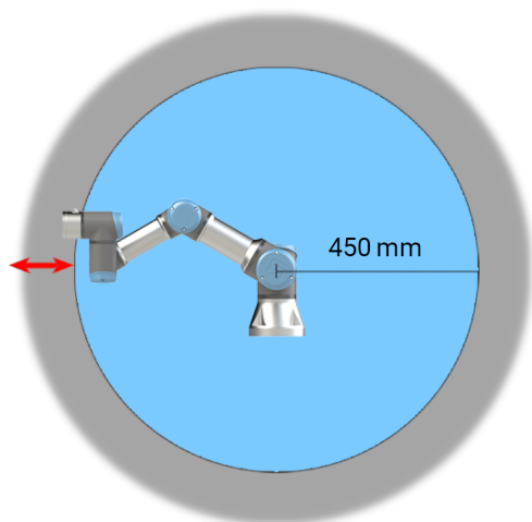
4.1: Zaradi fizičnih značilnosti robotove roke določena delovna območja terjajo pozornost na tveganje stiskanja. Eno območje (levo) je določeno za radialne premike, ko je člen zapetje 1 vsaj 450 mm od osnove robota. Drugo območje (desno) je znotraj 200 mm osnove robota, pri tangentsnem premikanju.
