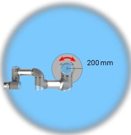
4.1: Zaradi fizičnih značilnosti robotove roke določena delovna območja terjajo pozornost na tveganje stiskanja. Eno območje (levo) je določeno za radialne premike, ko je člen zapetje 1 vsaj 450 mm od osnove robota. Drugo območje (desno) je znotraj 200 mm osnove robota, pri tangentsnem premikanju.
