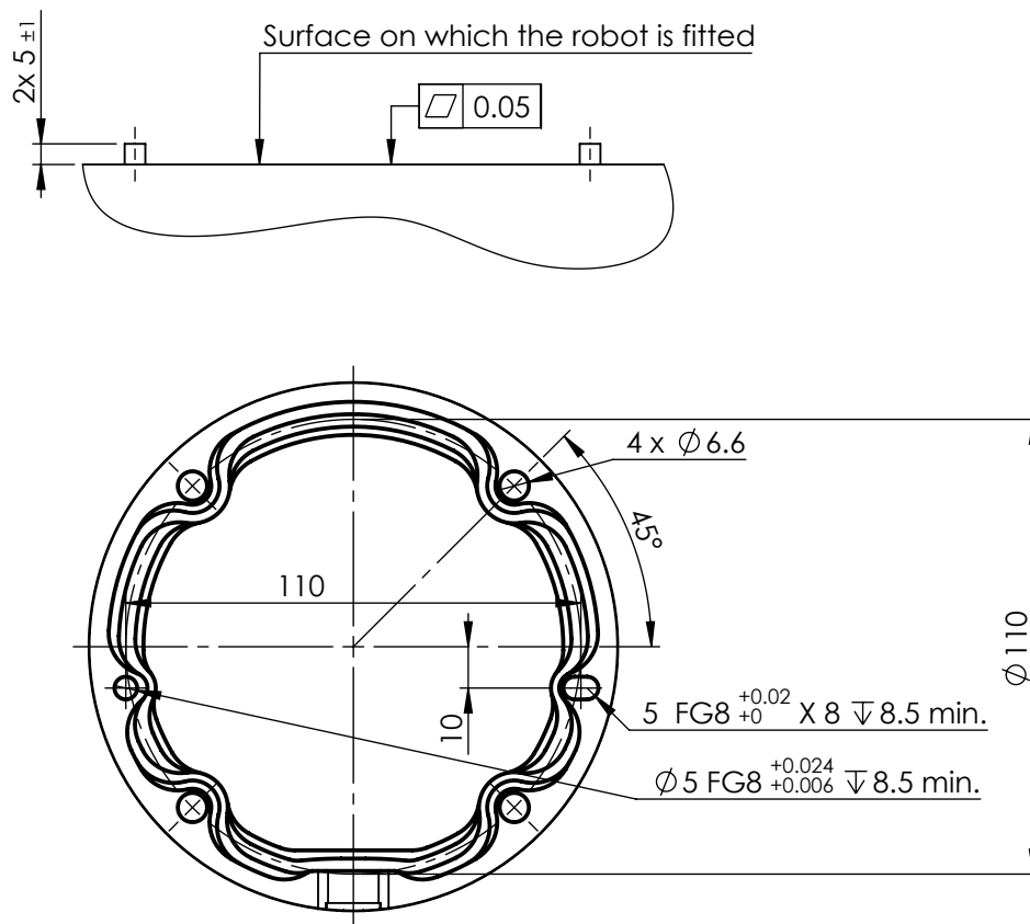
6.1: Odprtine za vgradnjo robota. Uporabite štiri vijake M6 . Vse mere so v mm .
