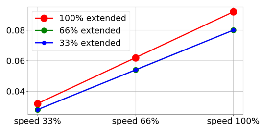
Čas ustavljanja v sekundah pri 66 % maksimalne obremenitve
