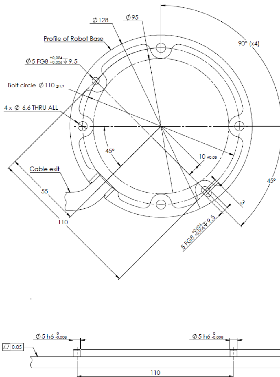
6.1: 机器人安装孔。使用四颗 M6 螺栓。所有测量值均以 mm 为单位。
