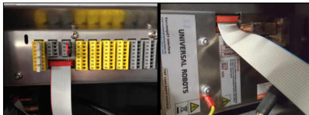
CF: 18.1: リボンケーブルの接続
