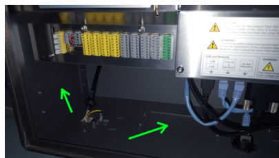
CF: 18.2: コントローラーボックス内のインターフェース配置
