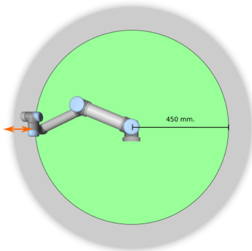
4.1: En determinadas zonas del espacio de trabajo debe prestarse atención a los peligros de enganche, debido a las propiedades físicas del brazo robótico. Se define una zona para movimientos radiales cuando la junta de la muñeca 1 está a una distancia de al menos 450 mm de la base del robot. La otra zona está a 200 mm de la base del robot, cuando el movimiento se produce en dirección tangencial.
