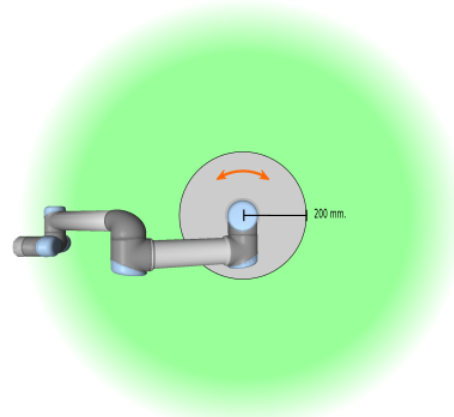
4.1: En determinadas zonas del espacio de trabajo debe prestarse atención a los peligros de enganche, debido a las propiedades físicas del brazo robótico. Se define una zona para movimientos radiales cuando la junta de la muñeca 1 está a una distancia de al menos 450 mm de la base del robot. La otra zona está a 200 mm de la base del robot, cuando el movimiento se produce en dirección tangencial.
