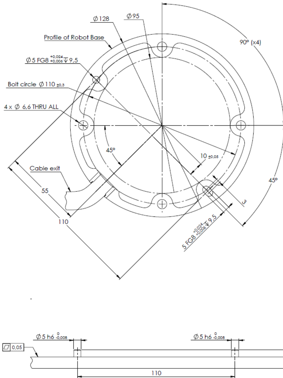
6.1: Orificios de montaje del robot. Use cuatro pernos M6 . Todas las medidas están en mm.
