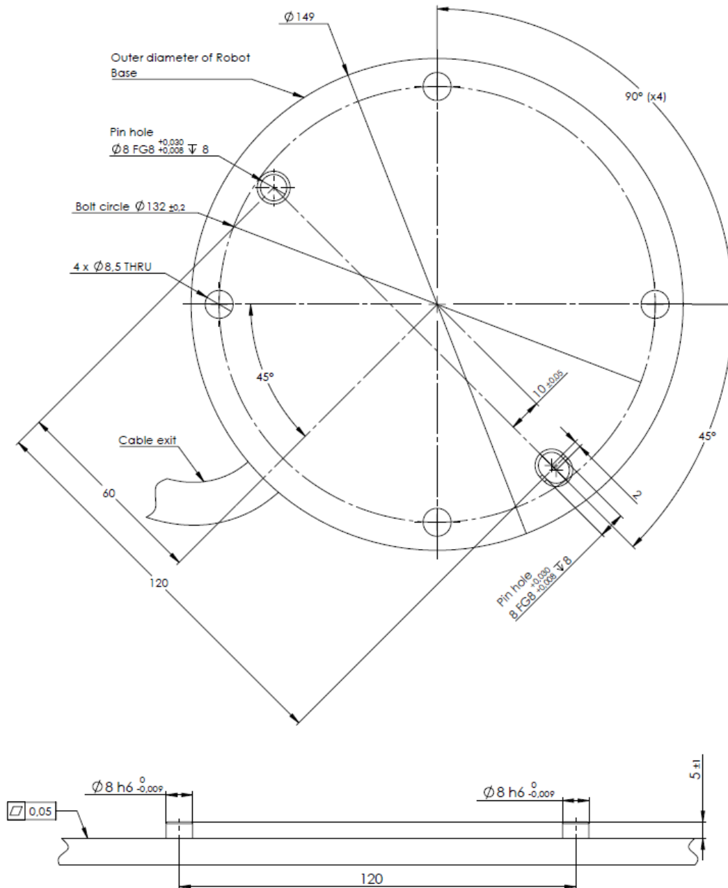
6.1: Orificios de montaje del robot. Use cuatro pernos M8 . Todas las medidas están en mm.
