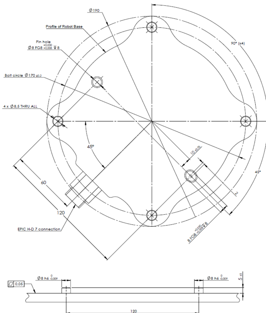
6.1: Huller til montering af robotten. Brug fire M8 bolte. Alle mål er i mm .
