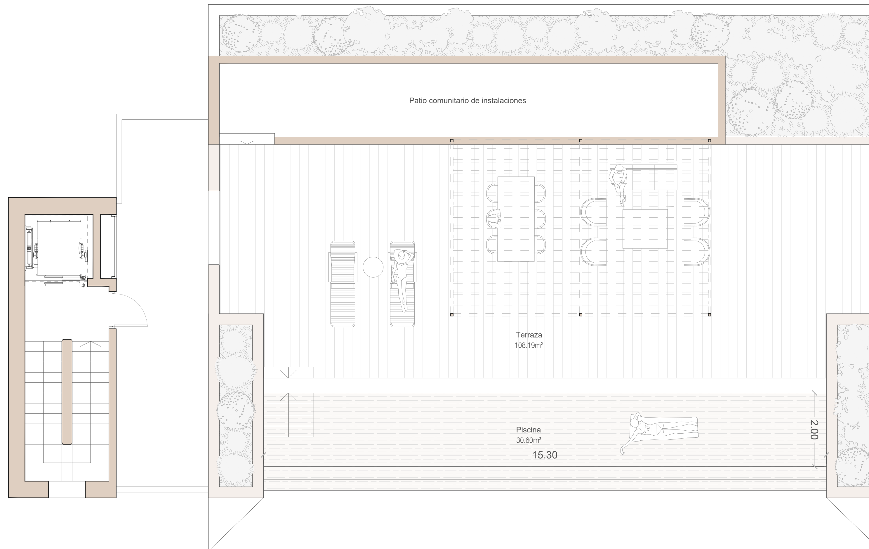
PLANTA ÁTICO PENTHOUSE FLOOR
