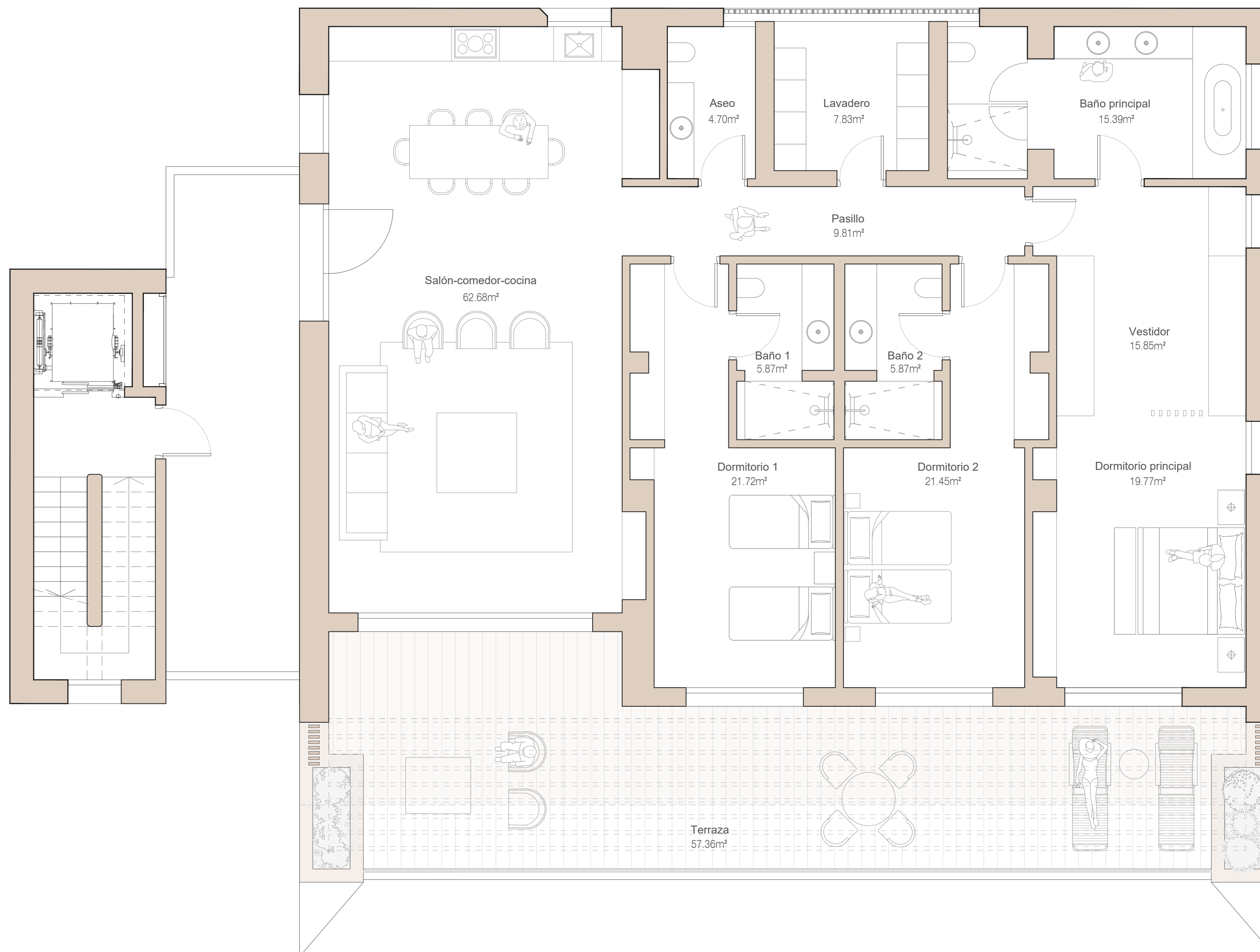
PLANTA CUARTA FOURTH FLOOR
