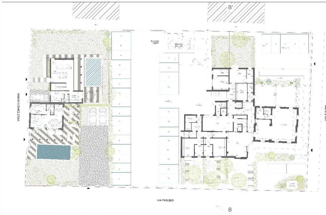
progetto HOTEL ARIANNA STATO DI PROGETTO Pianta piano terra studiolapis
