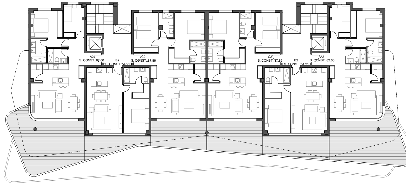
PLANTA 2ª
