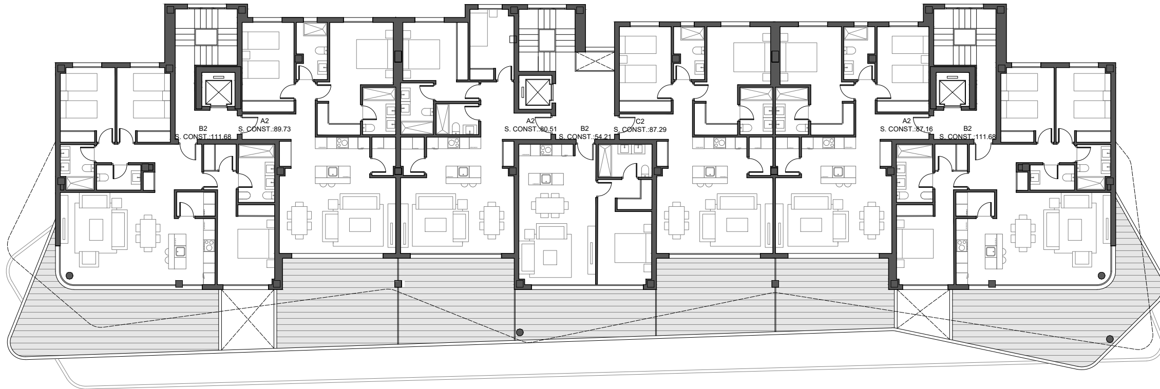
PLANTA 2ª
