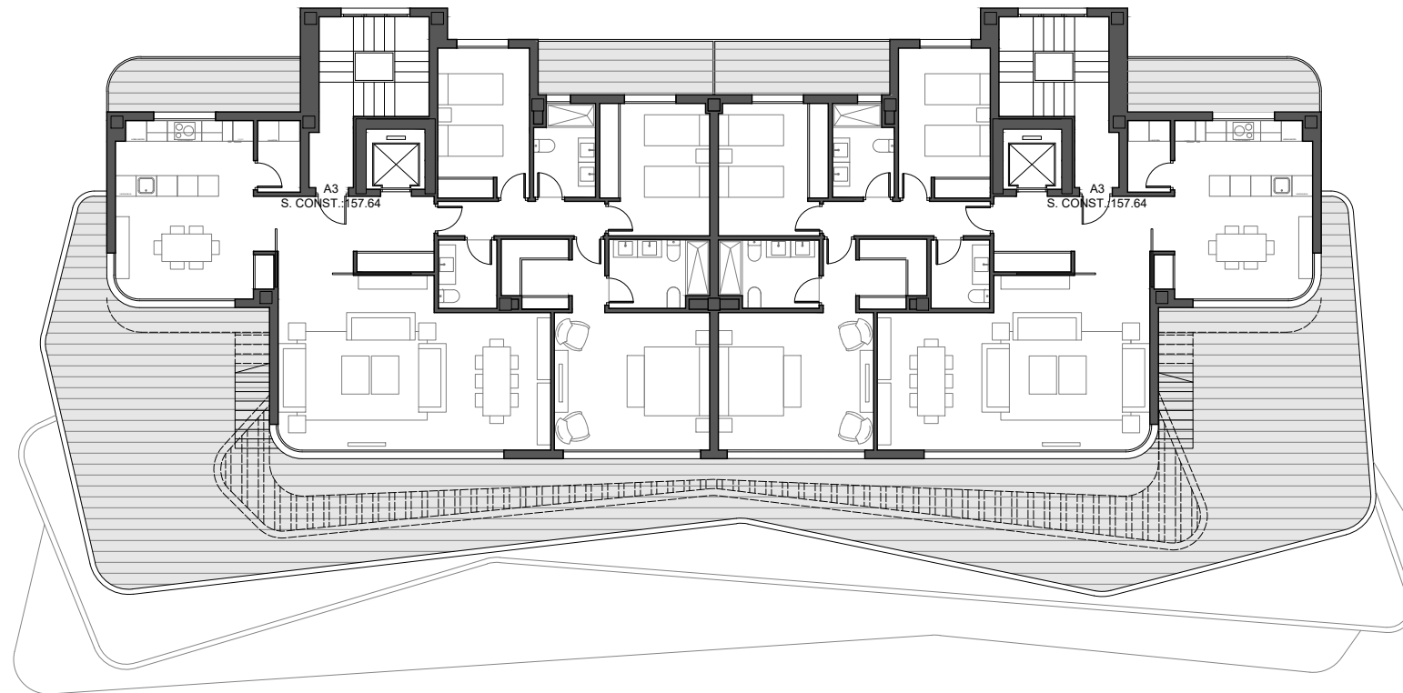
PLANTA 3ª
