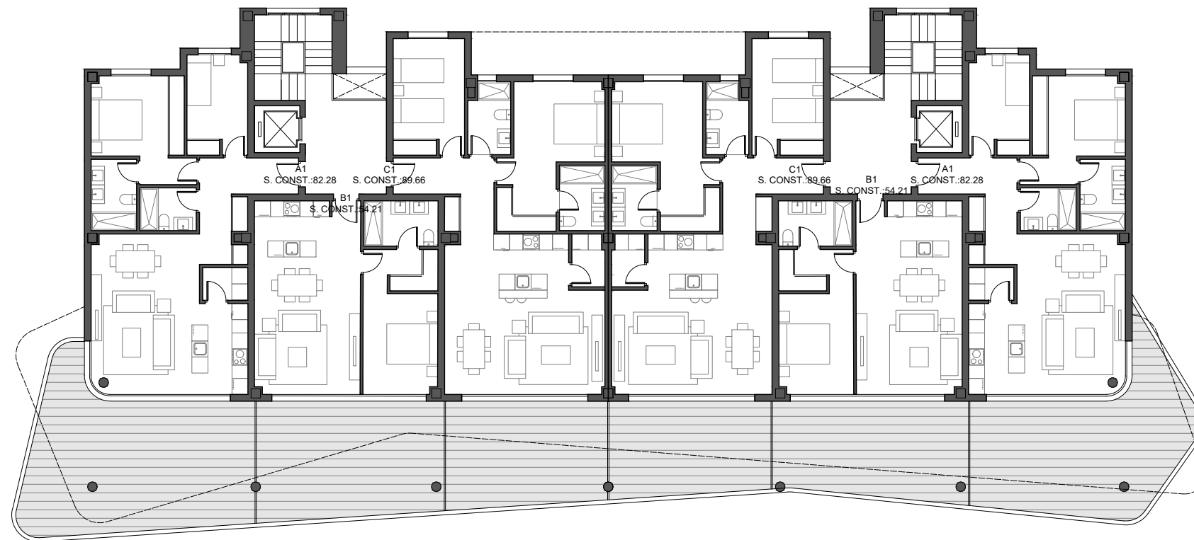
PLANTA 1ª
