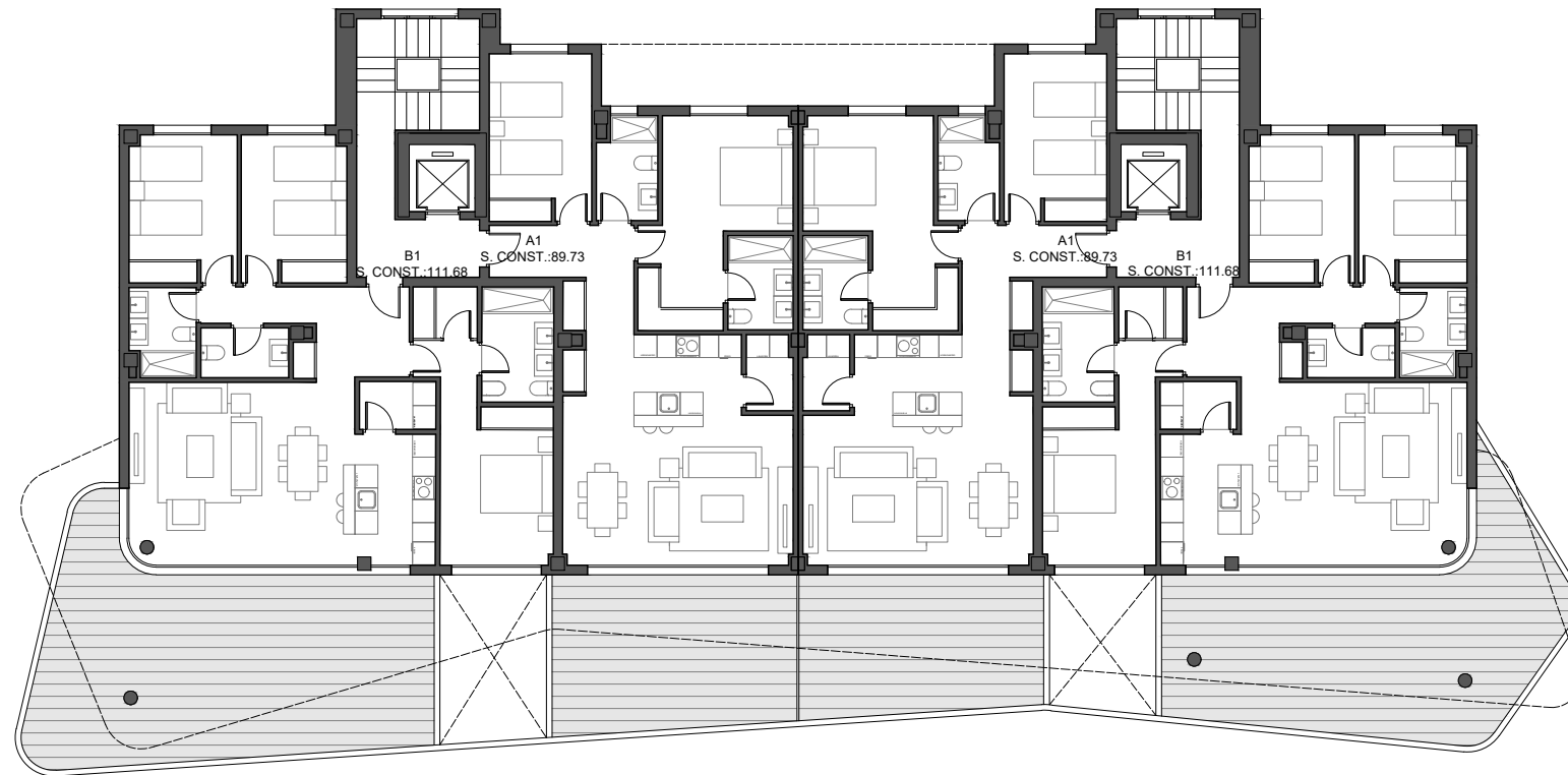
PLANTA 1ª
