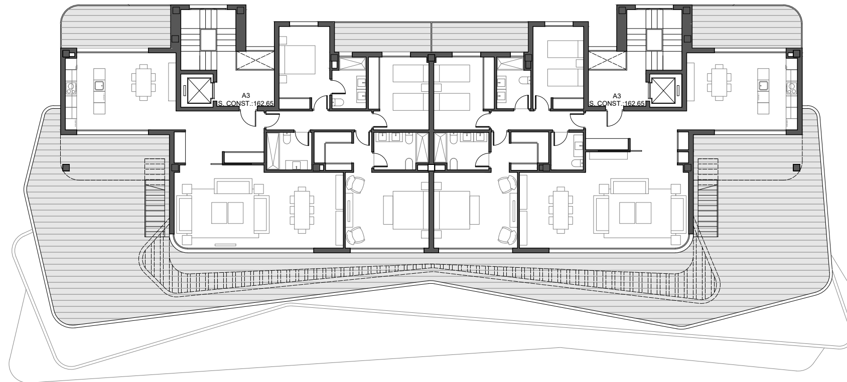
PLANTA 3ª
