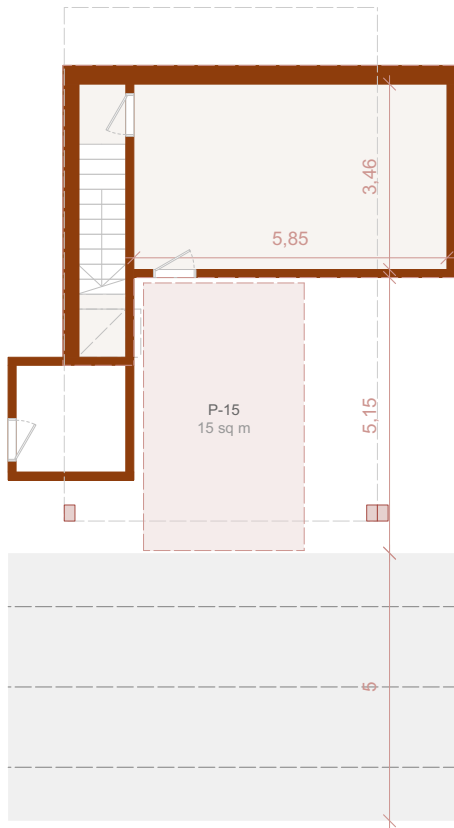
PLANTA SOTANO
