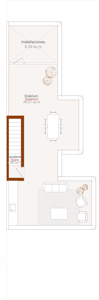
PLANTA CUBIERTA
