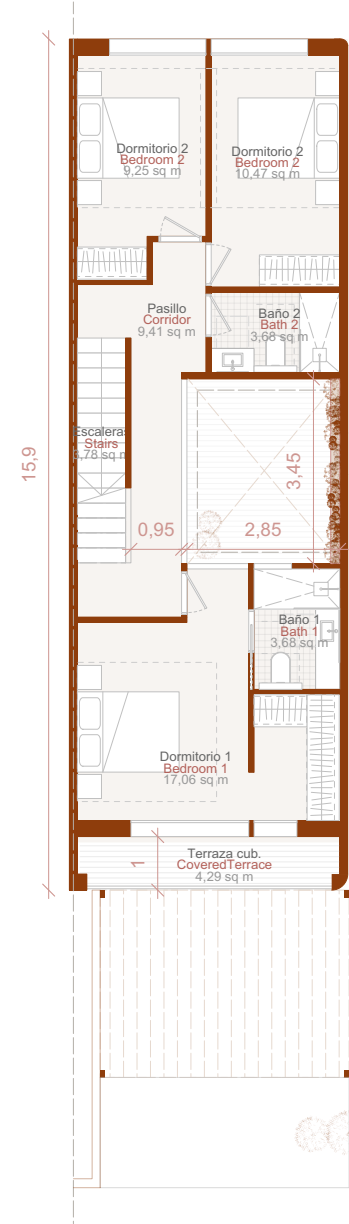
PLANTA PRIMERA
