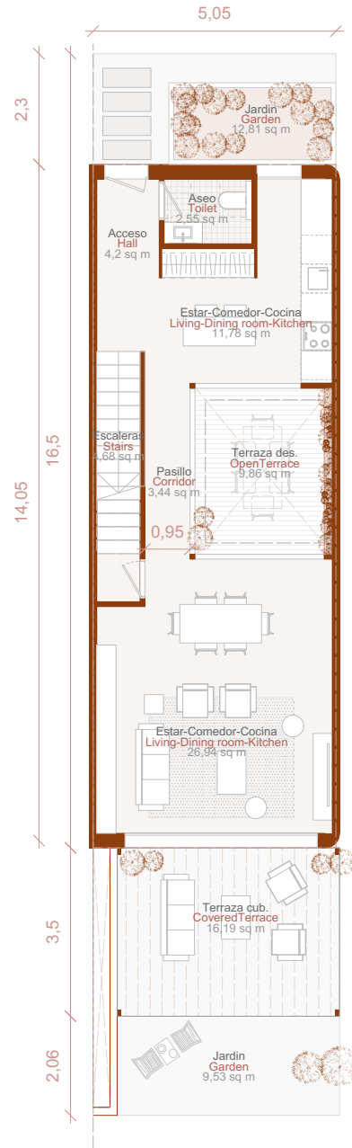
PLANTA BAJA
