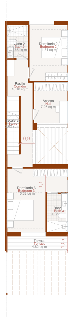
PLANTA PRIMERA
