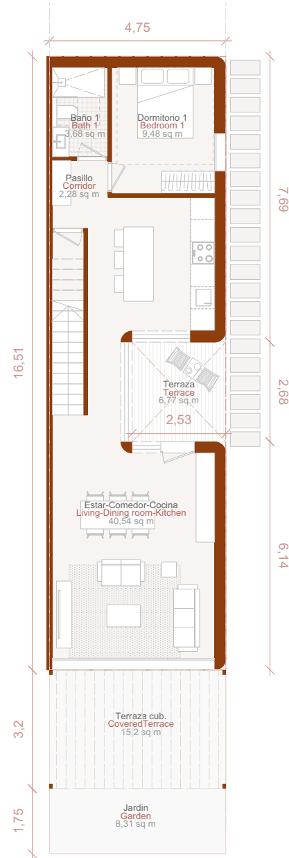
PLANTA BAJA
