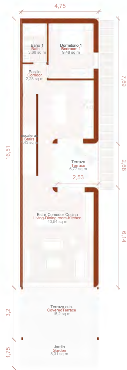
PLANTA BAJA
