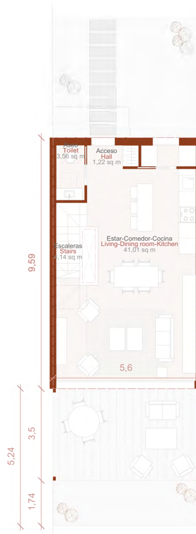
PLANTA BAJA
