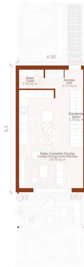
PLANTA BAJA
