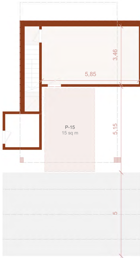
PLANTA SOTANO
