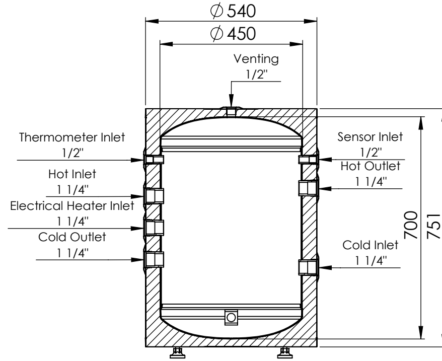
KESIT A-A
