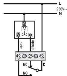
Collegamento ad una valvola motorizzata
