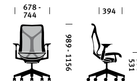
Seduta con schienale medio
