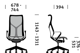
Seduta con schienale alto
