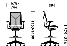
Sgabello con schienale medio
