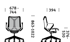
Seduta con schienale basso
