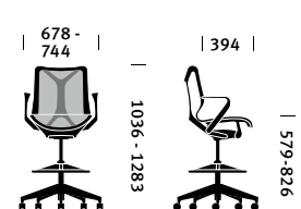
Sgabello con schienale basso
