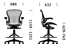
Sgabello con cilindro basso
