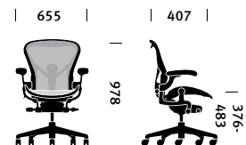
Seduta da lavoro Taglia A
