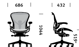
Seduta da lavoro Taglia B
