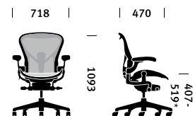
Seduta da lavoro Taglia C
