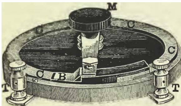
FIG. 118.—CARNOX RHEOSTAT.
