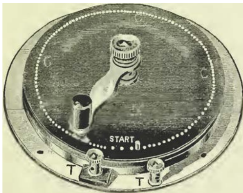
Fra. 119.-CA1<1.1ox RnEOSTAT.
