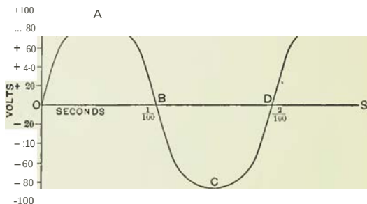
FIG. 44.—SINUSOIDAL ALTERNATING E. M. F.
