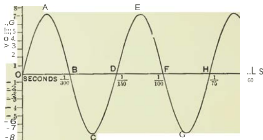
FIG. 49.-SINUSOIDAL E. M. F.
