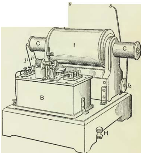
FIG. 141.-X-RAY APPARATUS.
