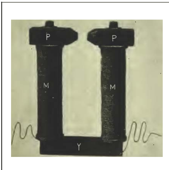
FIG. 81.—ELECTROMAGNET.
