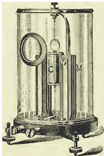
FIG. 38.-D'ARSONVAL GALVANOMETER.
