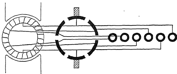
FIG. 122.—Leblanc's Panchahuteur.
