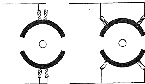
FIG. 92.—Double-brush rectifier.
