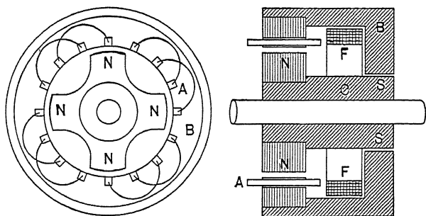
FIG. 136.—Inductor alternator.
